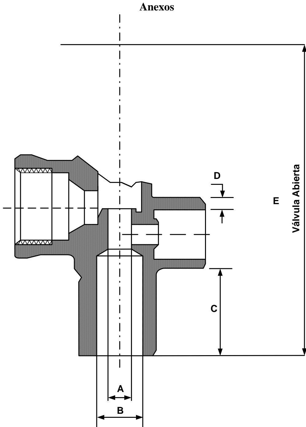
Figura No. 1.-Dimensiones de la válvula para recipientes portátiles Tipos I y II
