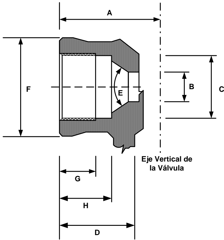
Figura No. 3.- Dimensiones de la conexión de salida
